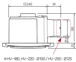
※HV-180, HV-220 : Ø100 / HV-250 : Ø125
