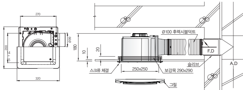
※HV-180, HV-220 : Ø100 / HV-250 : Ø125
